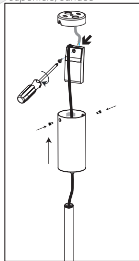
Tube 25 Superficie/Surface
